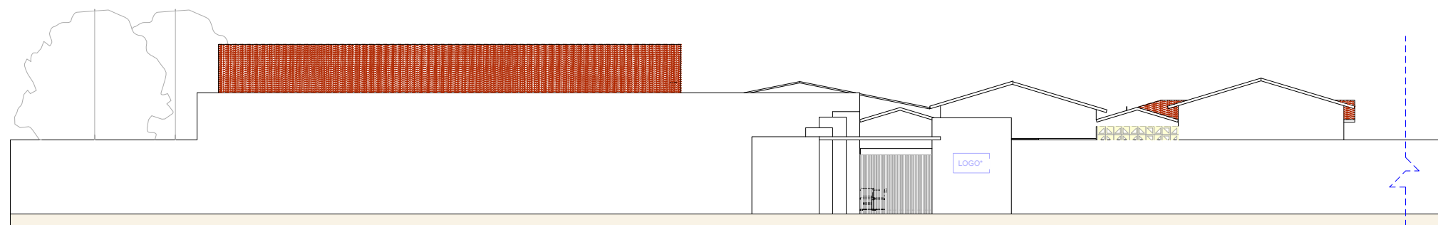
3 FRONTAL ESCALA 1:100
